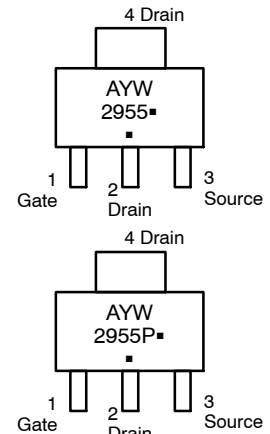
SOT-223 CASE 318E STYLE 3
